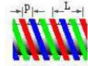
Filettatura a tre principi
