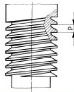
Profilo a dente di sega (buttress)
